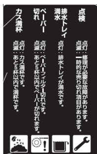
扉裏面の警告表示部
