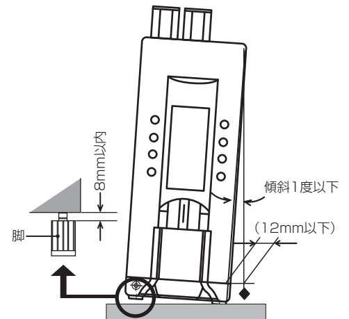
本機の傾き限界
